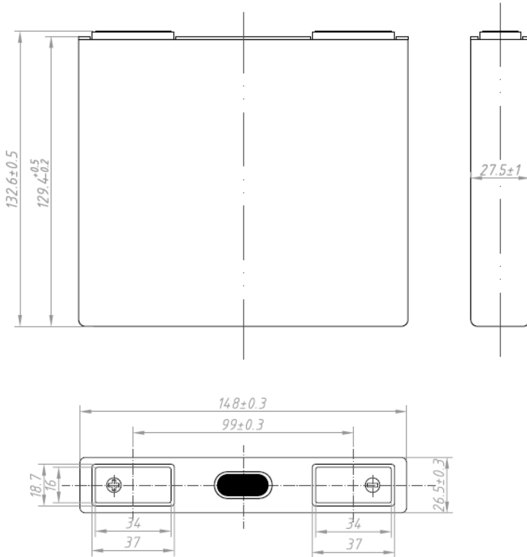
图 1 电池简易外形图
